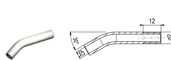
Prolunga per ugello di refrigerazione Cooling nozzle extensions
